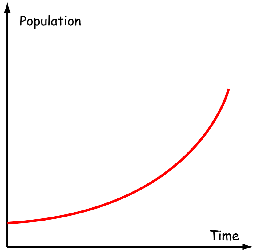
Function
