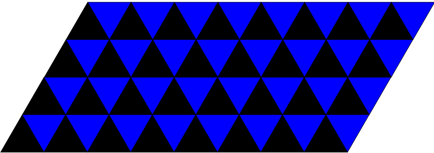
Tiling
