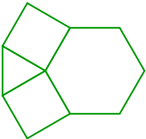
Vertex: 3.4.6.4
