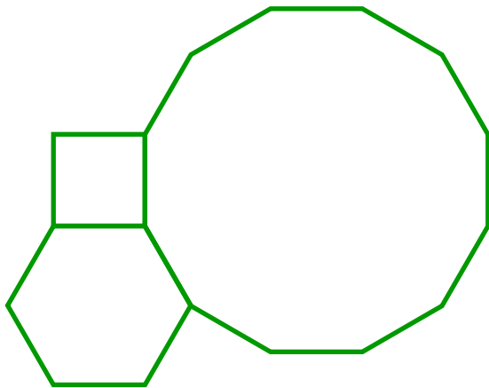
Vertex: 4.6.12
